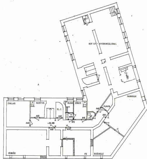
KÄLLARPLAN
